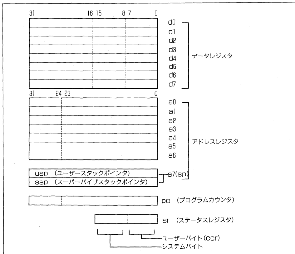
図1 68000のレジスタ
